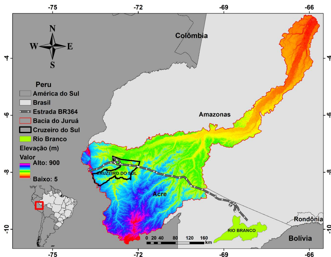
Figura 1. Localização geográfica da Bacia Hidrográfica do Rio Juruá, na Amazônia.
