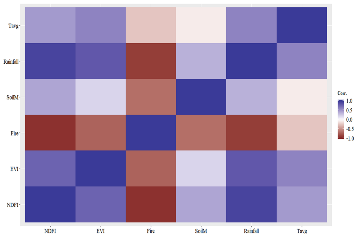
Figura 12. Matriz de correlação entre variáveis climáticas e ambientais para os anos de 2001 a 2018 na Bacia H. do Rio Juruá.
