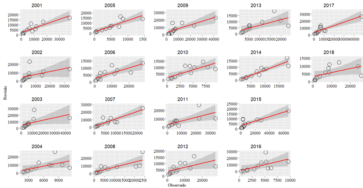
Figura 14. Análise de regressão dos dados observados e estimados do índice NDFI.
