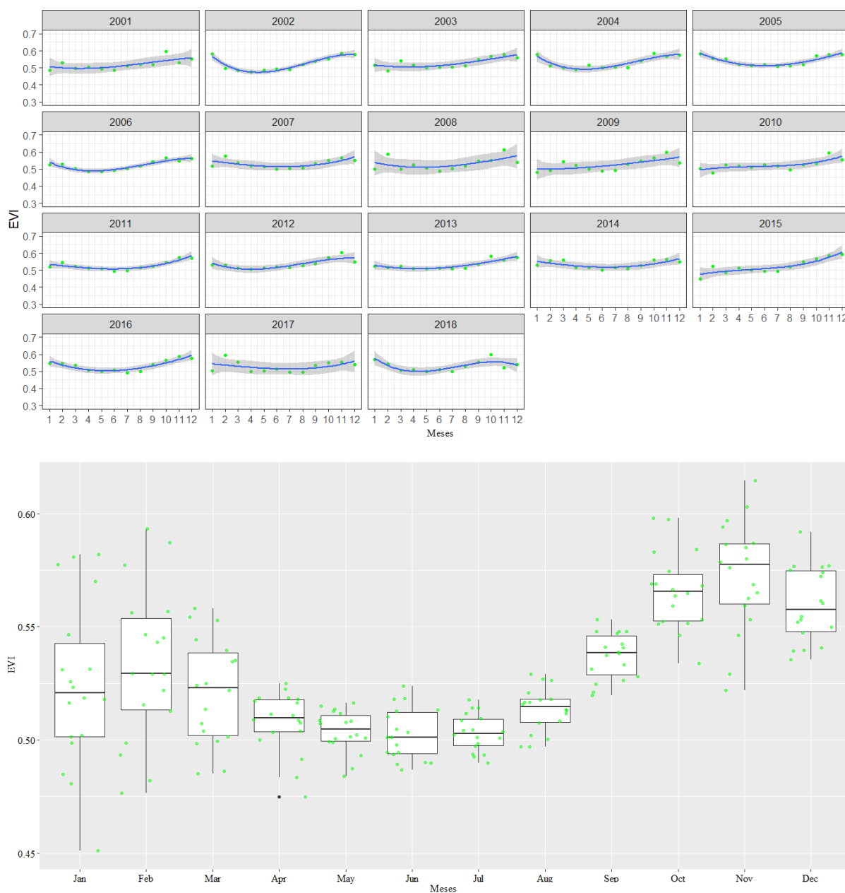
Figura 6. Valores mensais de EVI para a série de 2001 a 2018, na bacia Hidrográfica do Juruá.
