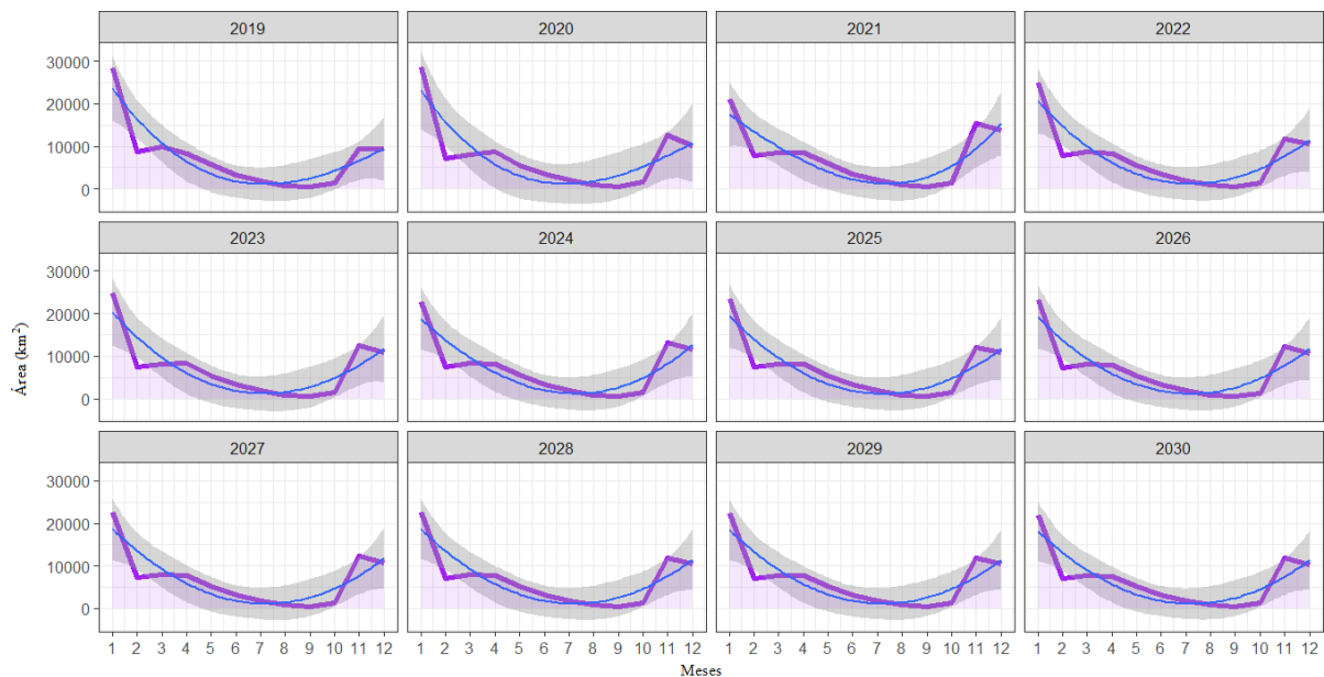
Figura 15. Modelagem futura do NDFI para a bacia do Rio Juruá.
