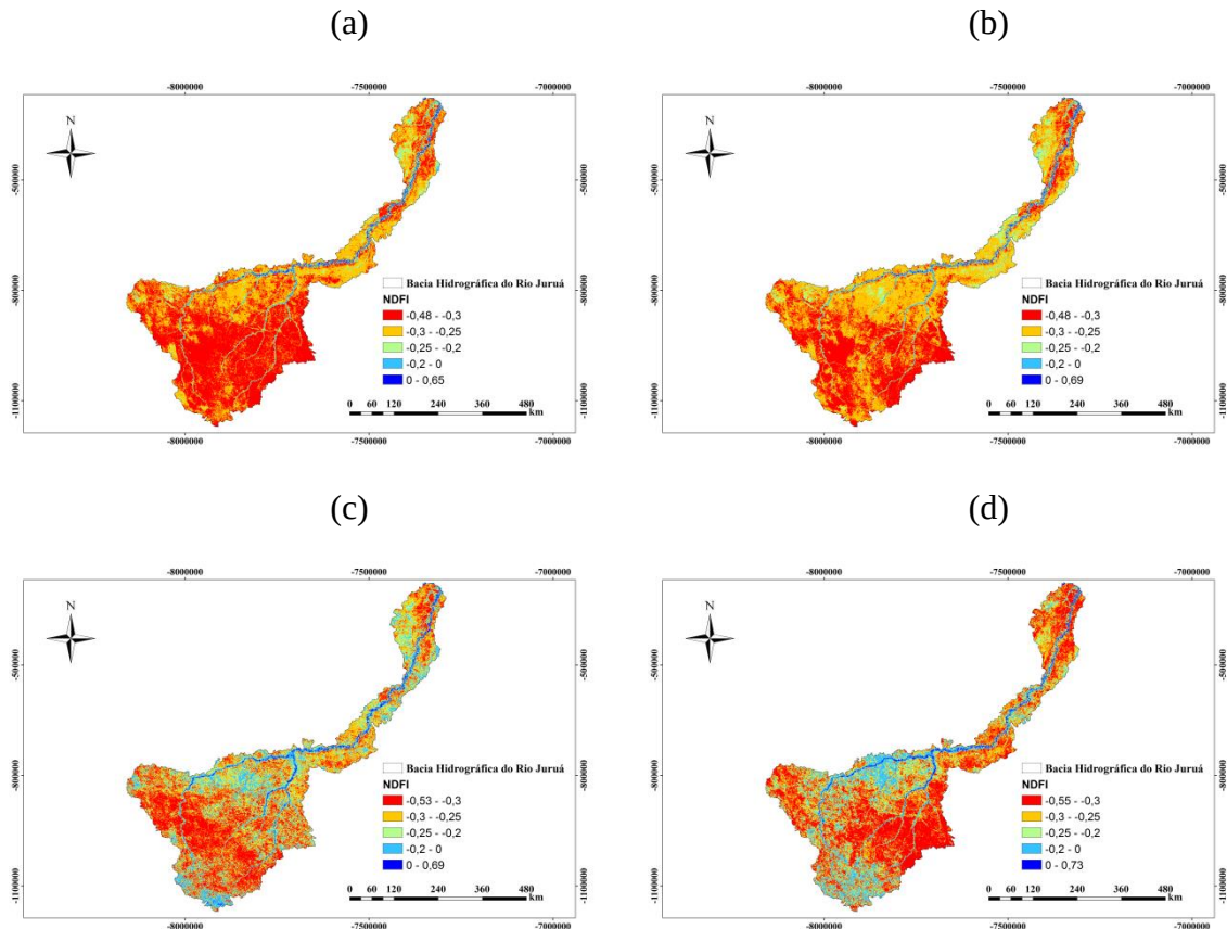
Figura 8. NDFI da bacia hidrográfica do Rio Juruá para os anos de 2005 (a) e 2010 (b) período seco, e os anos 2009 (c) e 2015 (d) período chuvoso.
