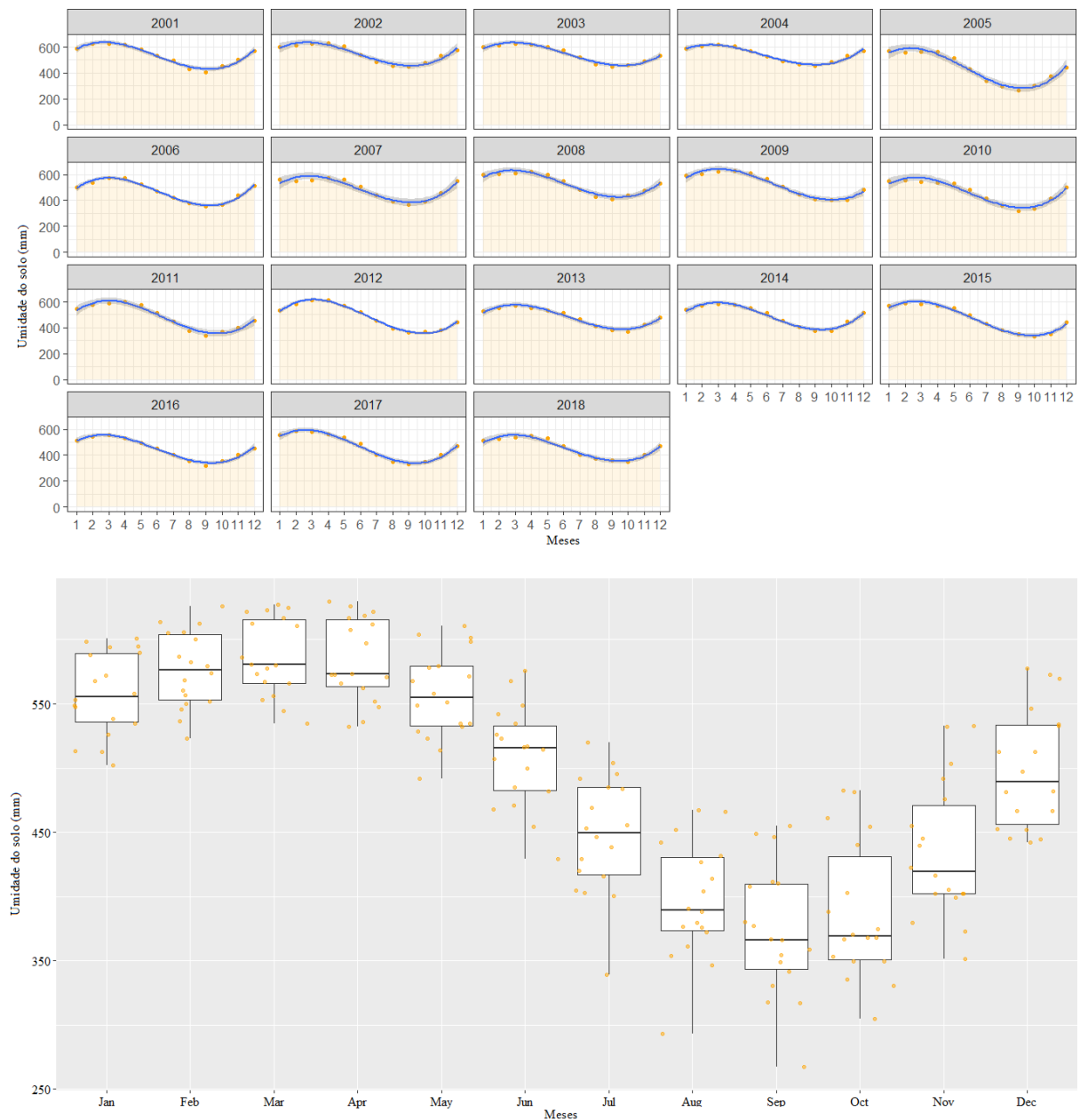
Figura 5. Umidade do solo mensal para a série de 2001 a 2018, na bacia Hidrográfica do Juruá.
