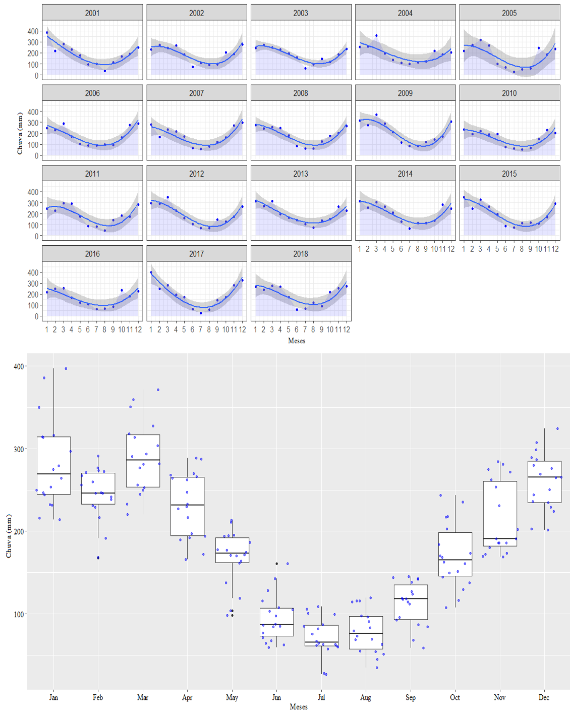
Figura 4. Chuva mensal para a série de 2001 a 2018, na bacia Hidrográfica do Juruá.
