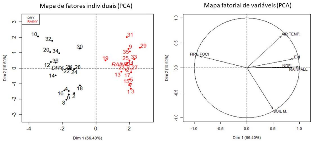
Figura 11. Mapa dos fatores individuais e das variáveis da ACP.
