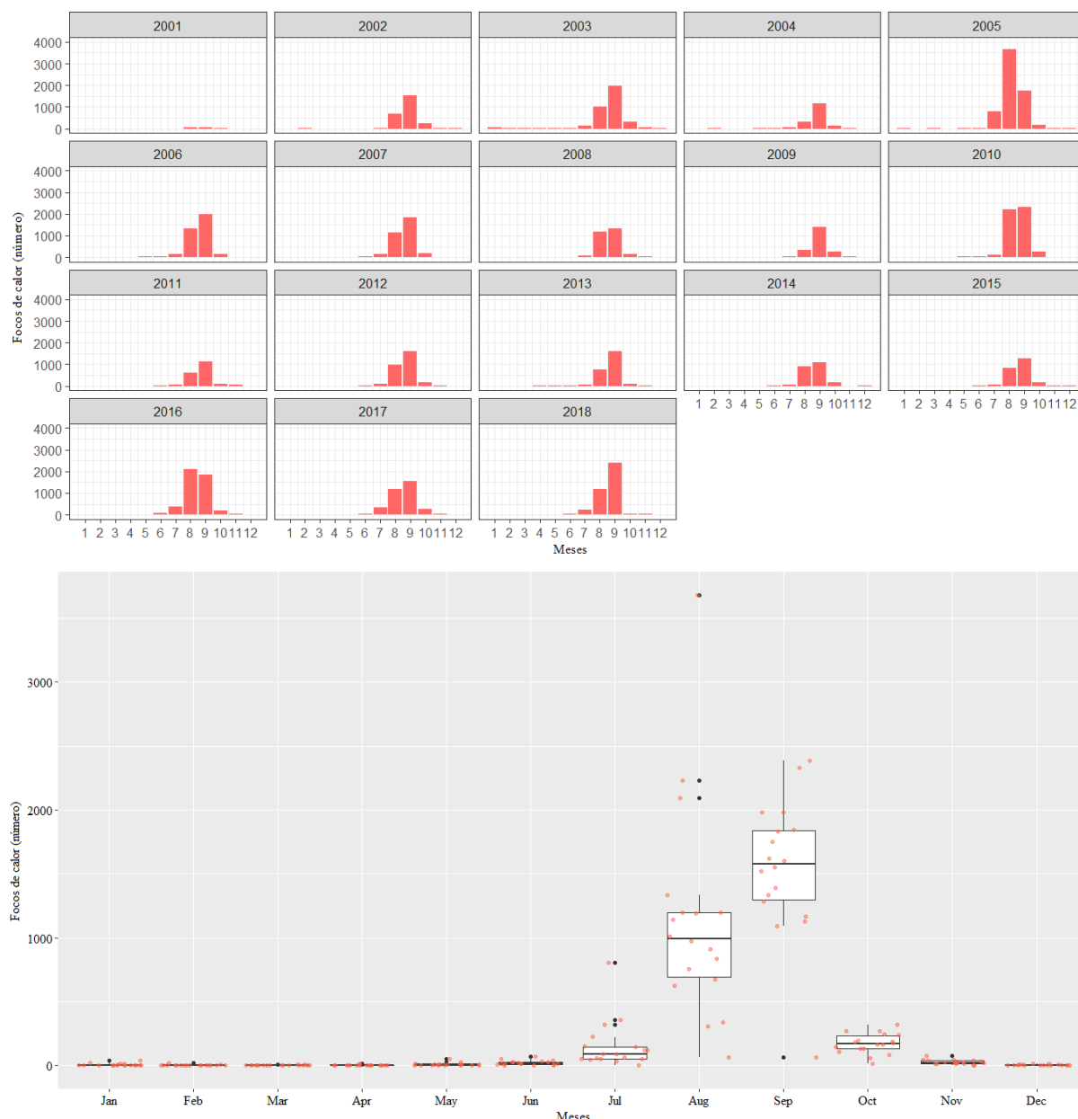
Figura 9. Distribuição mensal dos focos de calor para a série de 2001 a 2018, na bacia Hidrográfica do Juruá.
