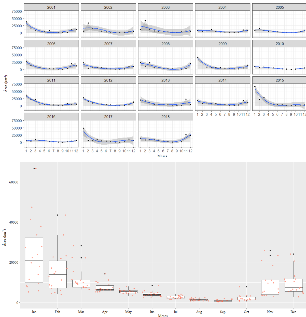
Figura 7. Valores de NDFI para a série de 2001 a 2018, na bacia Hidrográfica do Juruá.
